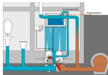
Extremfall: Kellerüberflutung
