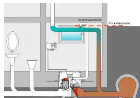
Notfall: Rückstau
