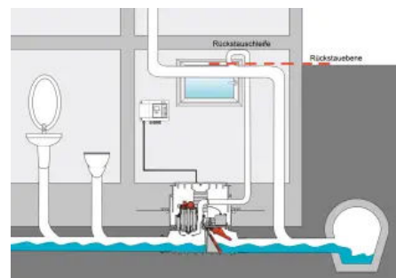
Normalbetrieb: Keller-Entwässerung
