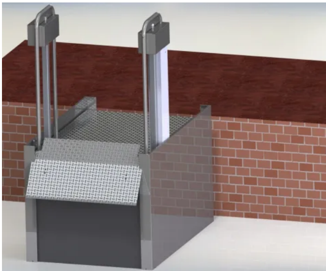
MB750 Micro A: Gerade Durchfahrt
