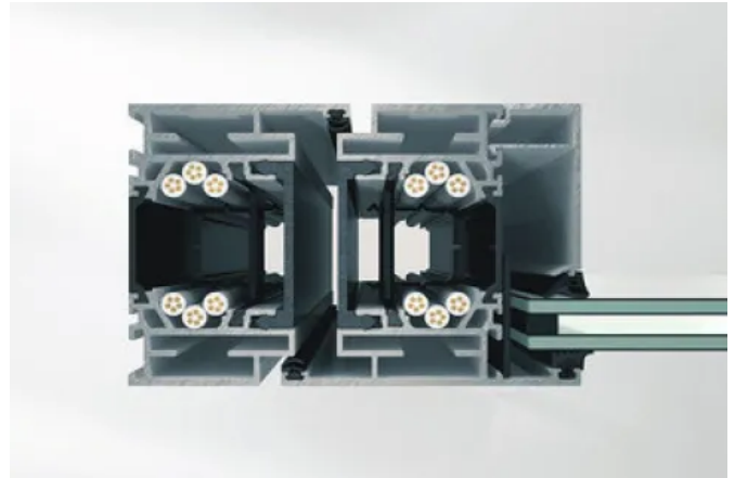
Falzzoffene Profilgeometrie
