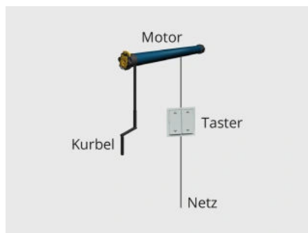
Basis: Steuerung über dezentrale Handbedienung „AUF/AB-Taster“ im Raum
