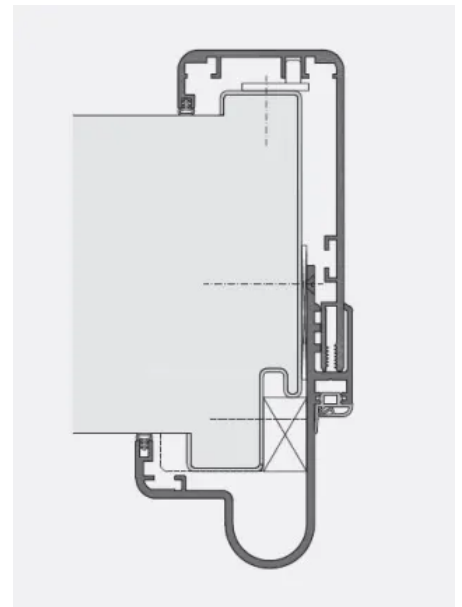
Zweischalige Umfassungszarge RENOFI mit Wanddickenausgleich | für stumpfe Türblätter und Fingerschutztüren
