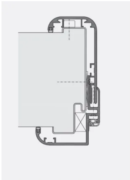
Zweischalige Umfassungszarge URFR mit Wanddickenausgleich | für Ganzglastüren sowie stumpfe und gefälzte Türblätter
