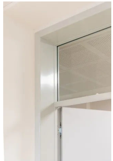
Aloys-Schreiber-Schule in Bühl | zweischalige Renovierungszarge RENOVI
