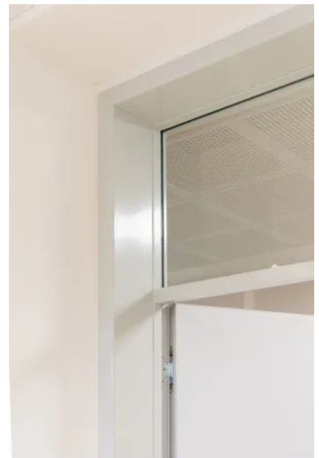
Aloys-Schreiber-Schule in Bühl | zweischalige Renovierungszarge RENOFI
