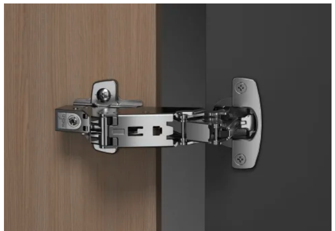
Sensys Weitwinkelscharnier
