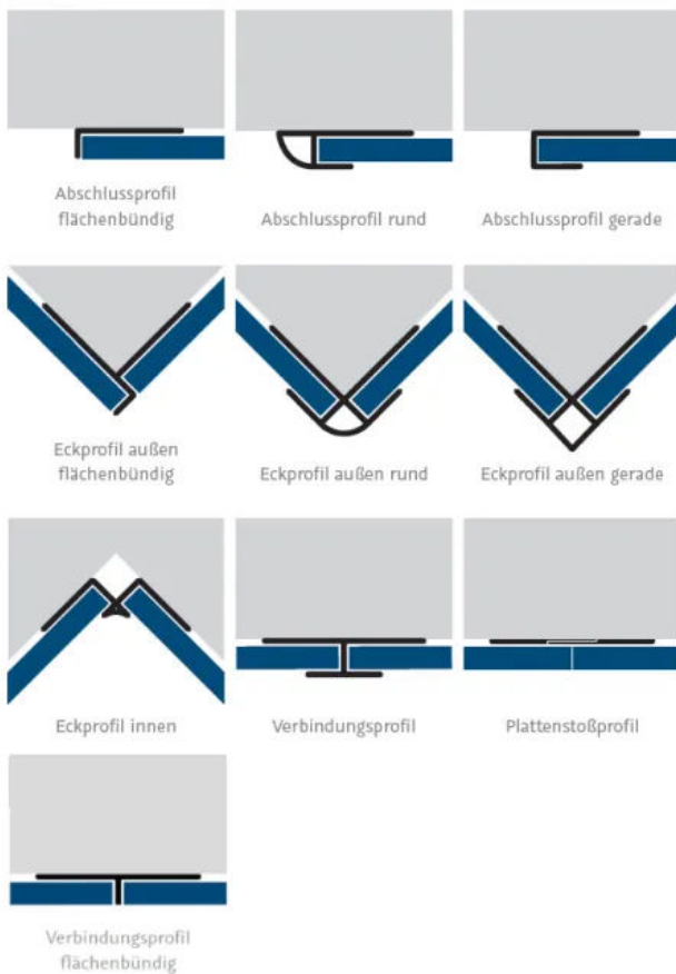
Plattenstoßprofil vor der Verbindung
