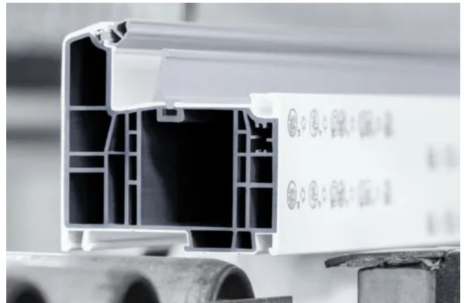
Einzigtartiges Extrusionsverfahren
