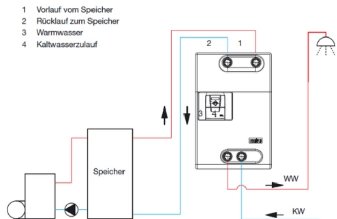
Schaltschema
