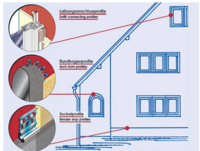
Mit speziellen Profilen für Laibungsanschlüsse, Rundbögen und Sockel bietet Protektor für jede Situation das passende Putzprofil.
