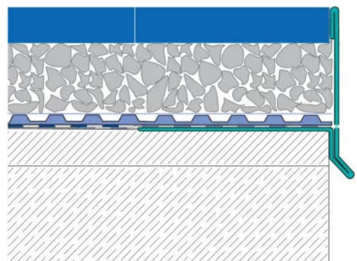
BLANKE_BALKON-KIESLEISTE Schnitt
