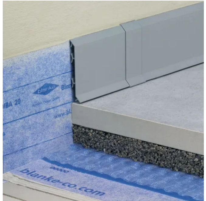
BLANKE BALKON-SOCKELBLENDPROFIL
