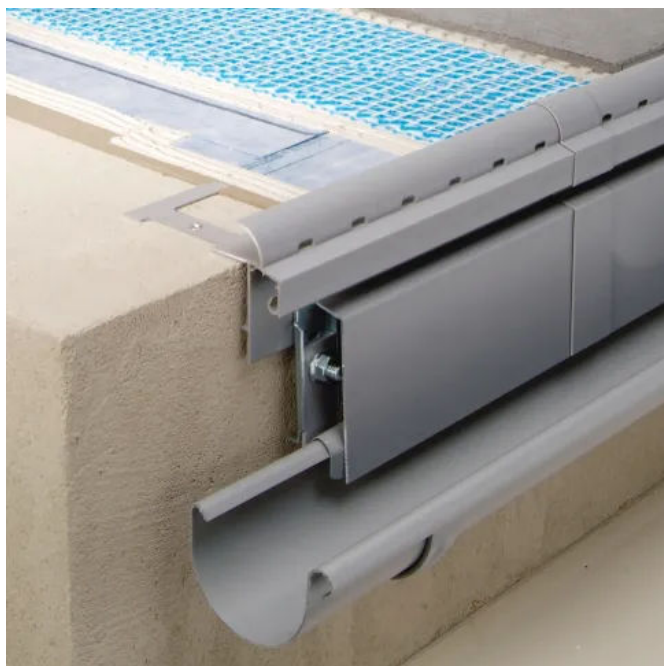
BLANKE BALKON-DRAINVIERTELKREIS / RINSYS-R
