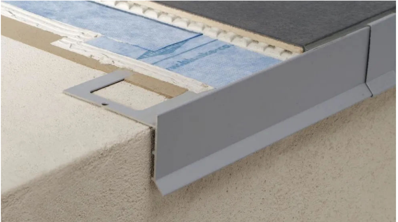
BLANKE BALKON-ABSCHLUSSWINKEL
