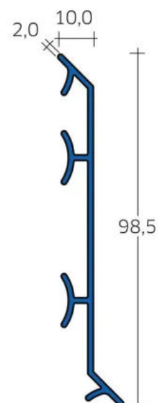
BLANKE BALKON-SOCKELBLENDPROFIL, technische Zeichnung
