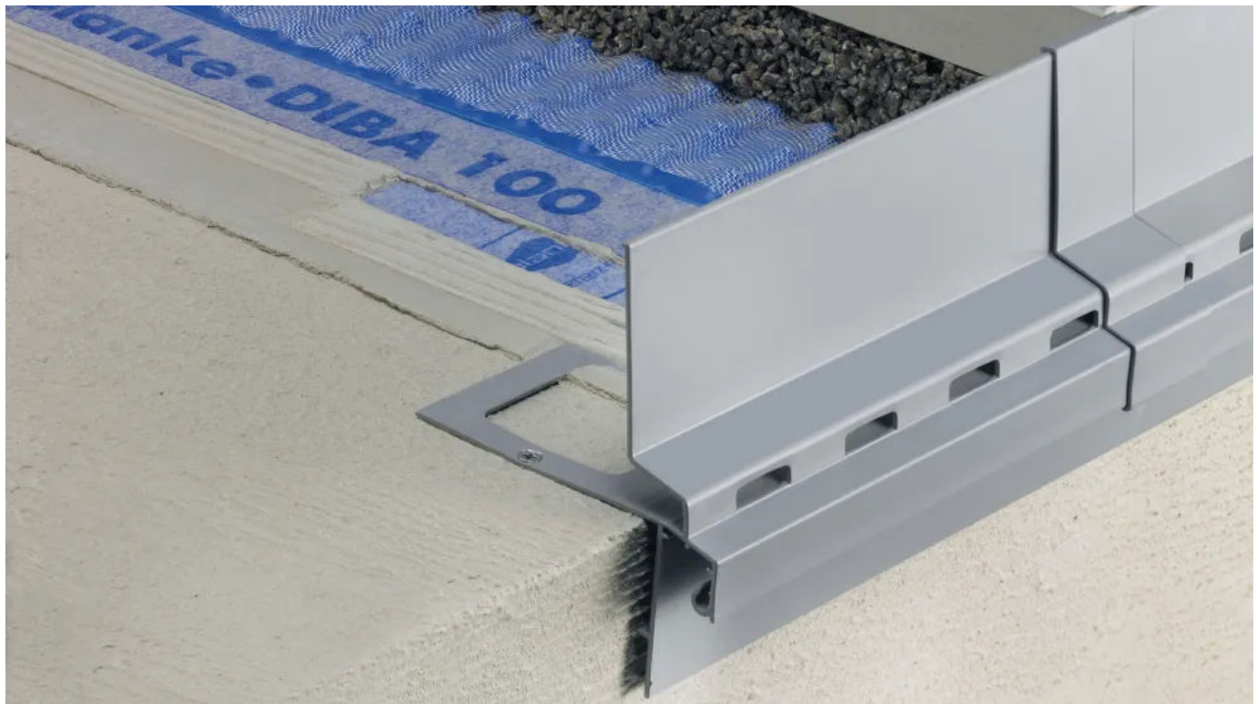
BLANKE BALKON-DRAINKIESLEISTE
