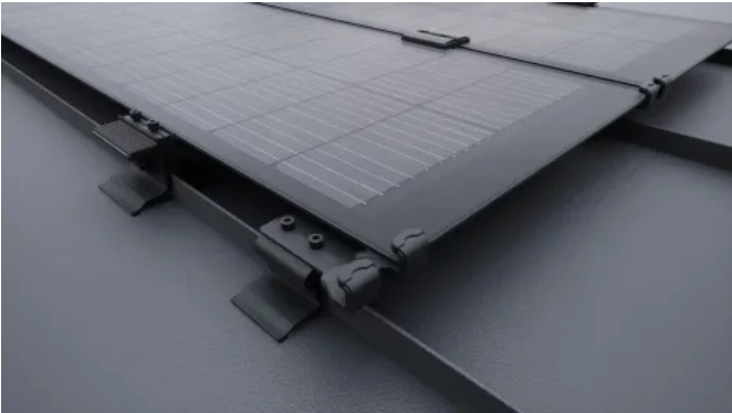
Falz- und Modulklemme in einem Produkt, einfache und schnelle Montage durch wenig benötigte Komponenten
