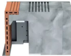
Ziegel-Raffstorekasten Poroton-RSK
