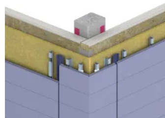
Außenecke als Ekelement – Planum waagrecht auf Kassetten-Innenschale mit vorgesetzter Dämmung
