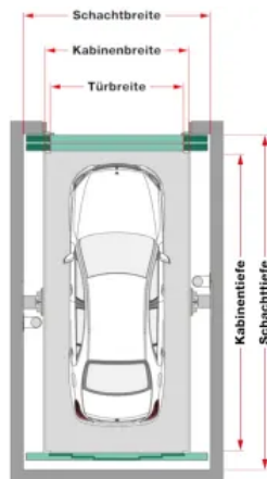
Schacht-, Kabinen- und Türmaße
