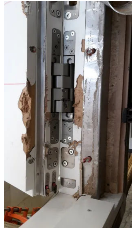
Das „PIVOTA® DXS 300 3-D“ weist eine Tragfähigkeit von 350 Kilogramm pro Paar auf und besteht ausschließlich aus Stahl. Dadurch erreicht das Band die Einbruchhemmung der Widerstandsklasse RC4. Das Bild zeigt das Band nach bestandener Einbruchprüfung. Foto: Huber Form Schreinerei GmbH, Triftern-Neukirchen
