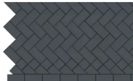
Fischgrätverband, Anschluss mit halben und angeschnittenen Pflasterklinkern
