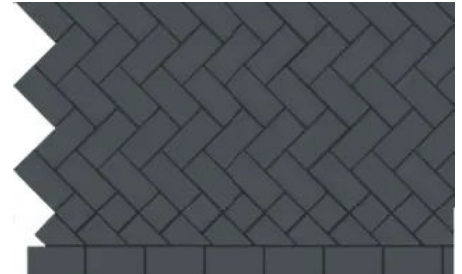
Fischgrätverband, Anschluss mit halben und angeschnittenen Pflasterklinkern
