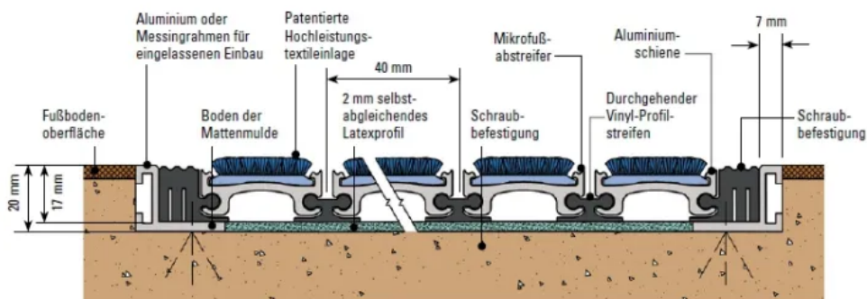
Aufbau Pedisystems (Beispiel Pediluxe®)
