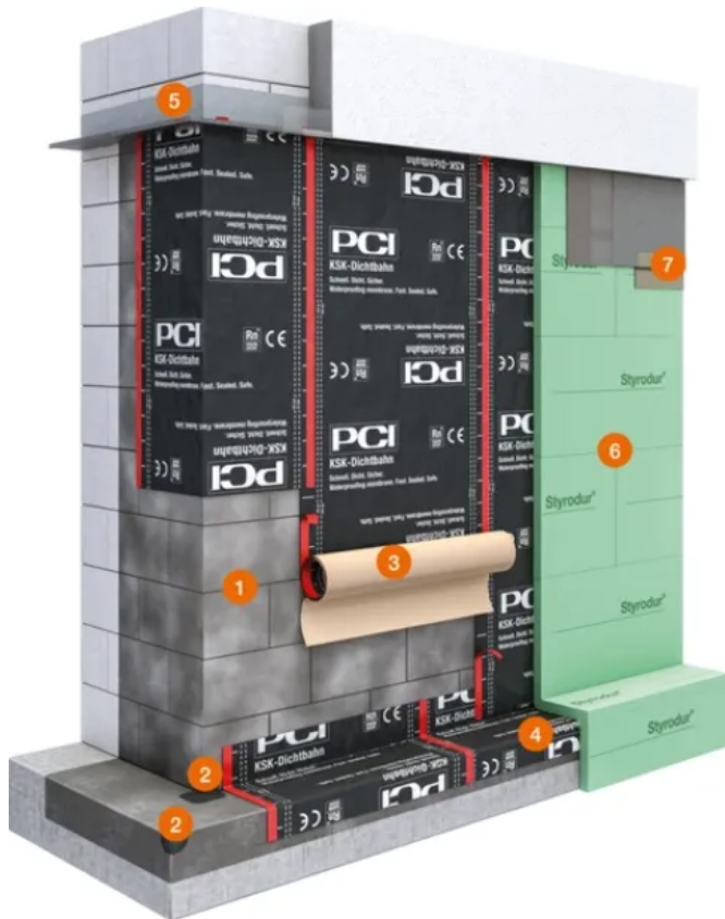
Bauwerksabdichtung KSK (kaltselfstklebende Bitumen-Dichtbahn)
