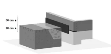
W 4-E – Spritzwasser, Sockelbereich
