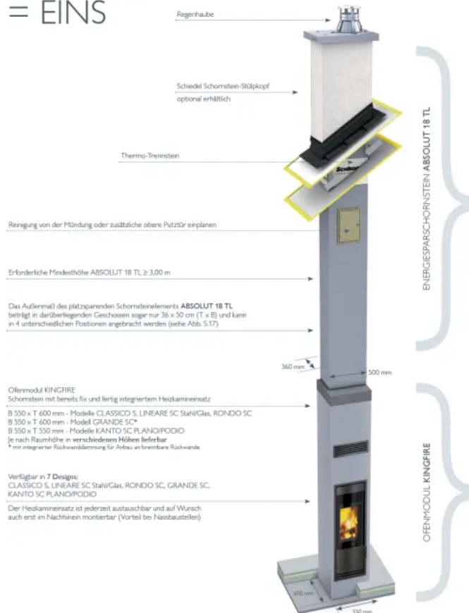
KINGFIRE Systemaufbau
