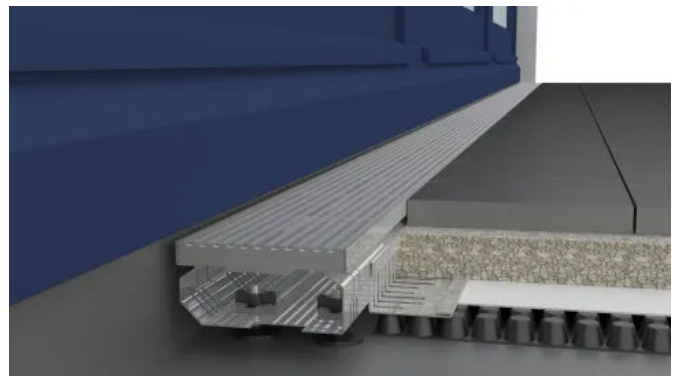
MONSUN® DRAINTEC Entwässerungsrinne höhenverstellbar - Baubreite 100, 125, 155, 200, 250 mm
