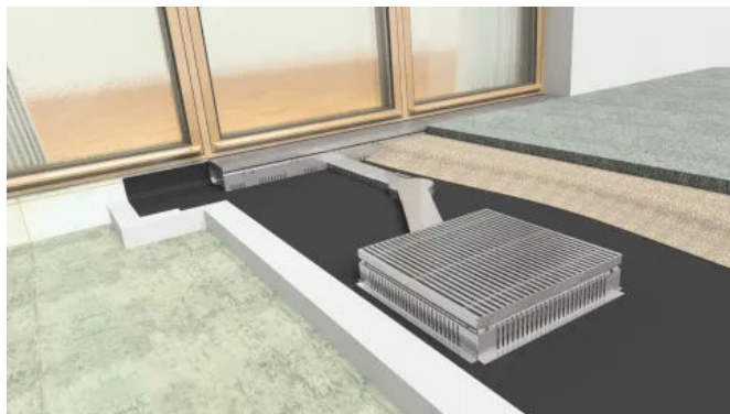
MONSUN® Terrassenbausatz für die zuverlässige und flexible Anpassung der Entwässerung an den Terrassenaufbau
