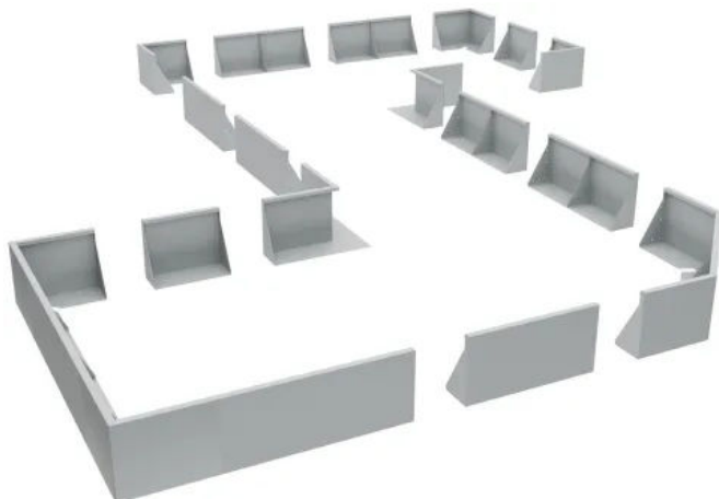
MONSUN® GALA Systembauteile
