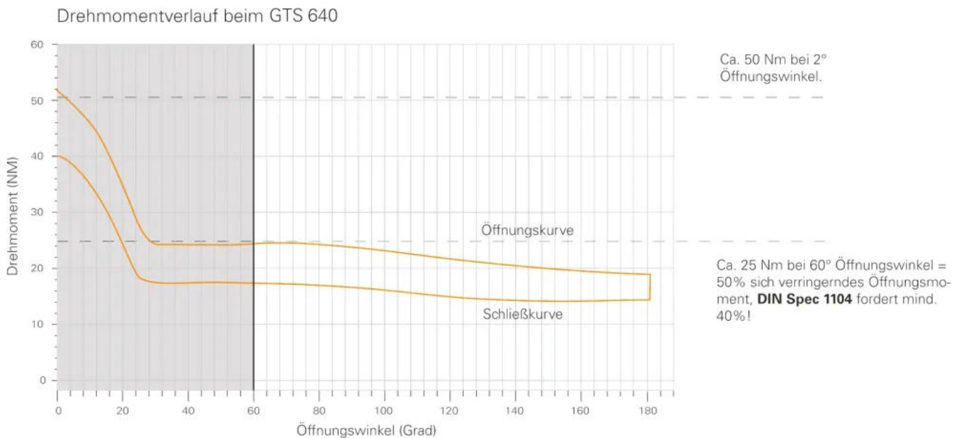
Drehmomentenverlauf Obentürschließer GTS 640
