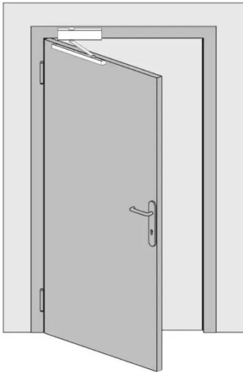
Beispiel für Kopfmontage Bandseite DIN L
