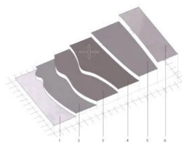
Nuvolato Architop® Estrichboden – Systemaufbau
