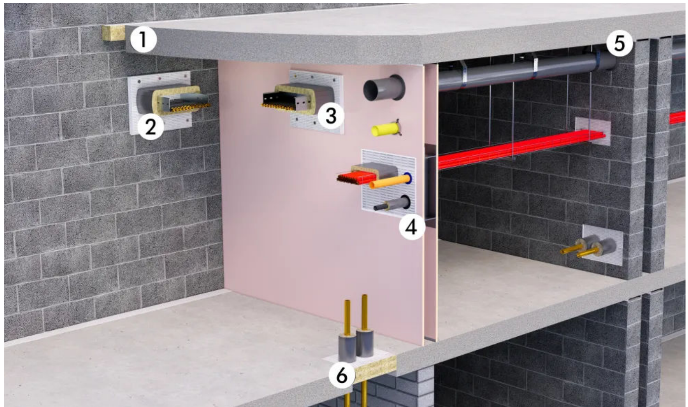
Systeme und Lösungen für verschiedenste Brandschutzanforderungen in Bauteilfugen sowie zur Abschottung von Rohr-, Kabel- und Elektrodurchführungen in Wänden und Decken.
