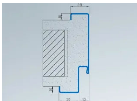
Umfassungszarge Profil 23 | Ruck-Zuck-Anker
