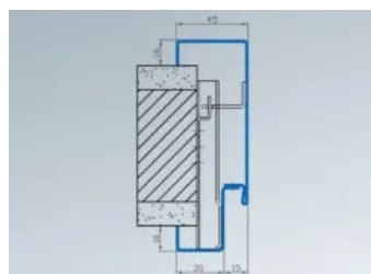
2-teilige Steckzarge Profil 2140 für alle Wandarten
