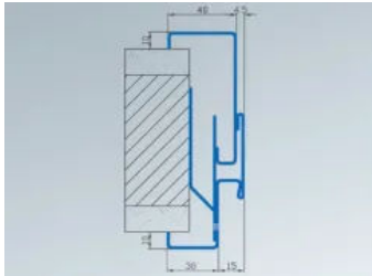
2-teilige Steckzarge Profil 2150 mit Maulweitentoleranz für Mauerwerk
