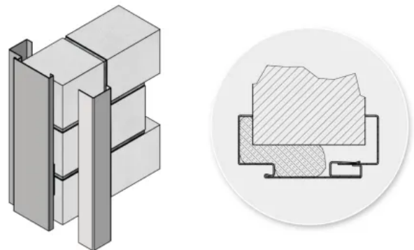
UniFix Light | 3D-Darstellung und Querschnitt
