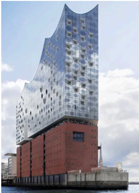
Elbphilharmonie | 2-flügelige Stahlrahmentür System Fuego light T30-2 RS als Brandabschluss
