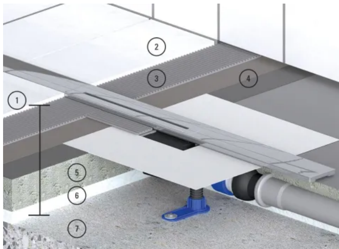
Die Aufbauhöhe setzt sich zusammen aus Estrich + Wärmedämmung + Abdichtung + Kleber + Oberbelag
