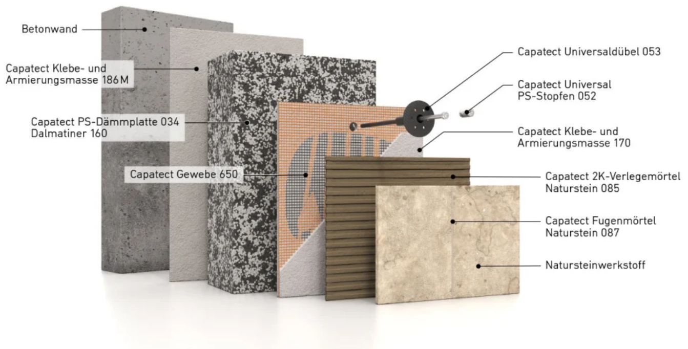
Beispielhafter Systembau
