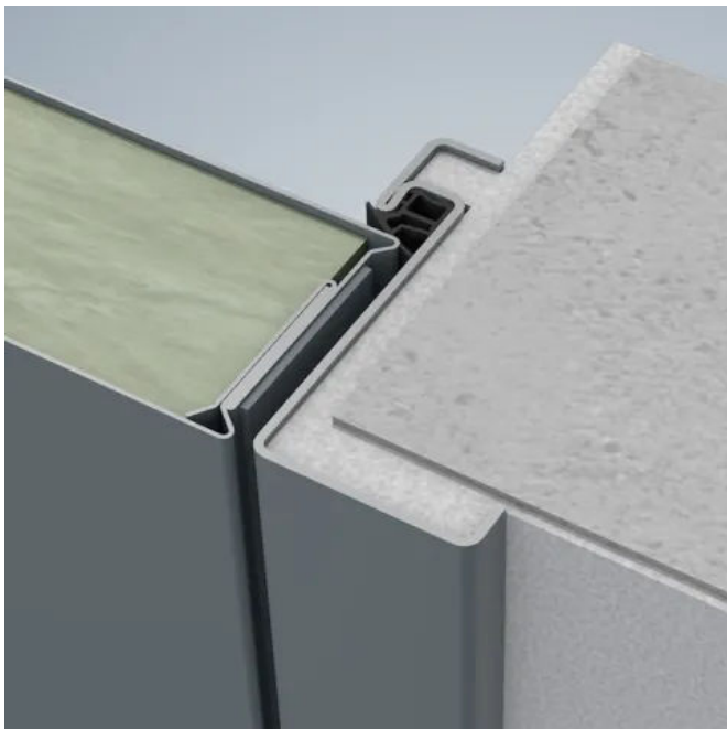
NovoPorta Plano | Der stumpfe Türeinschlag
