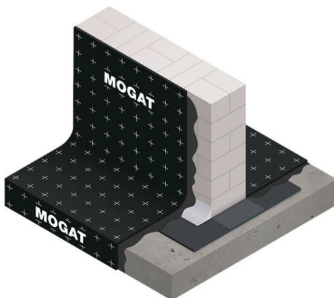
Abdichtung Kelleraußenwand
