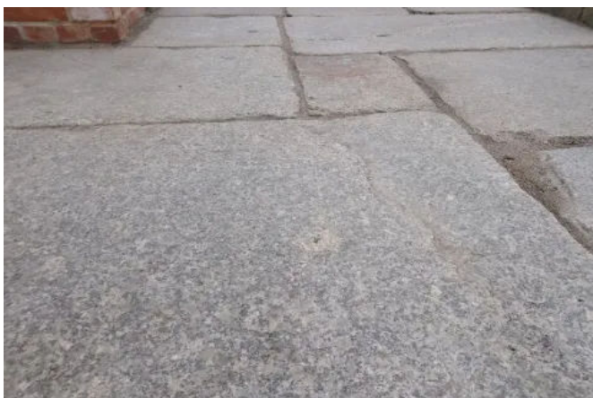
ReUse Krustenplatte 15-30cm Stärke
