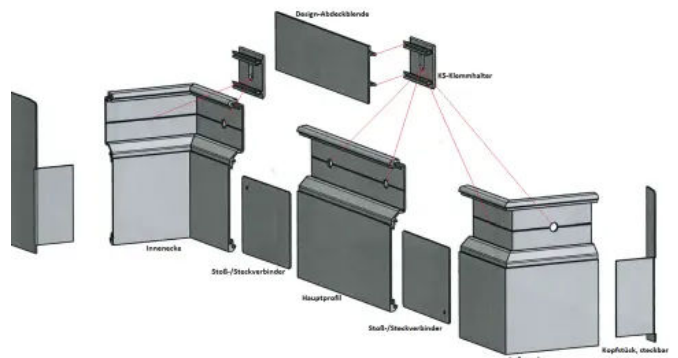
Systembauteile TWAP Connect
