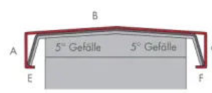
Attika-/Mauerabdeckung 5 Kanten, beids. Gefälle, PM-5
