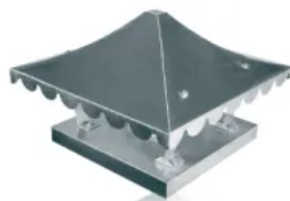
Kaminhaube Typ 10 Sauerland, Kupfer o. Edelstahl 1,5 mm
