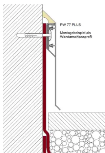
Terrassenwandanschluss- / Trittschutzprofilssystem TWAP DESIGN
