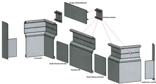
Systembauteile TWAP Connect
