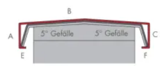
Attika-/Mauerabdeckung 5 Kanten, beids. Gefälle, PM-5
