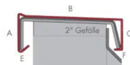
Attika-/Mauerabdeckung 5 Kanten, PM-2
