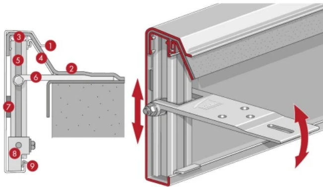
Flachdachabschluss Flex
