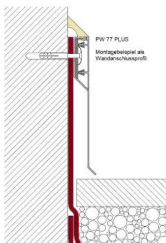
Terrassenwandanschluss- / Trittschutzprofilsystem TWAP DESIGN
