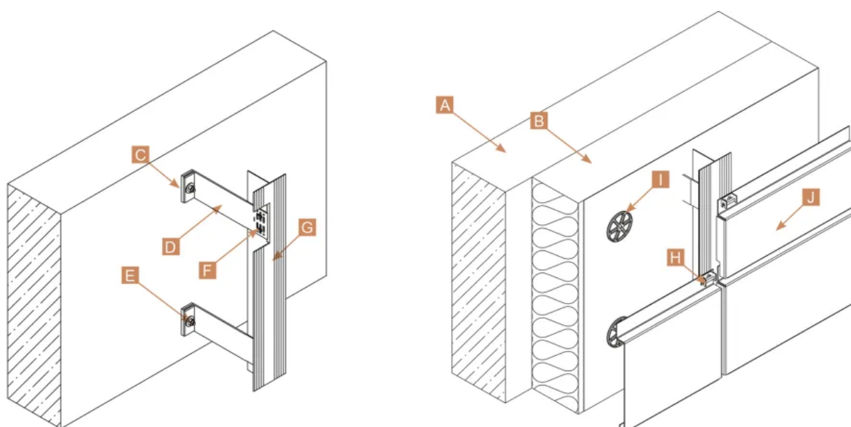
KFM BASIC Detail Kreuzpunkt
