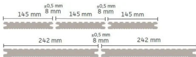
Profilskizze
