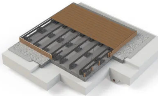
Terrassenaufbau mit VARIO FIX II und Konstruktionsbalken
