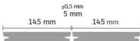
Profilskizze
