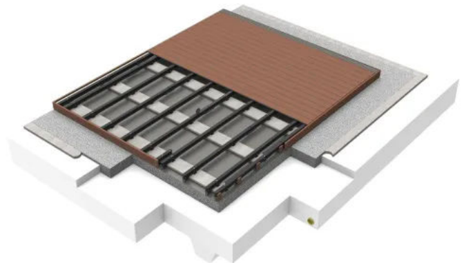
Terrassenaufbau mit Betonrandsteinen und Konstruktionsbalken
