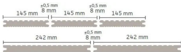
Profilskizze
