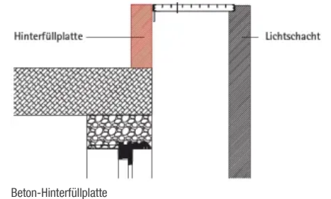
Beton-Hinterfüllplatte
