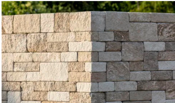
GDM.DECA wall, proActive Set 20 und Set 10, antikplus, Muschel-Kalk nuanciert, proClean 100
