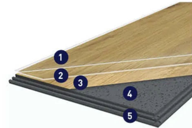
Vinyl-Objektfliesten CREATION 70 MEGACLIC | Produktaufbau
