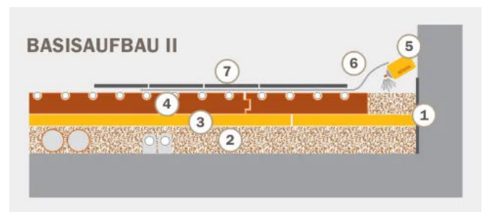
Basisaufbau für geklebte Bodenbeläge
