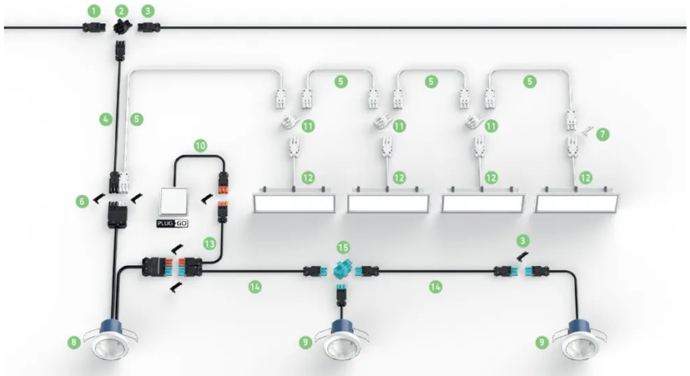
Systemverkabelung für Theben Präsenz- und Bewegungsmelder mit gesis®-Anschluss
