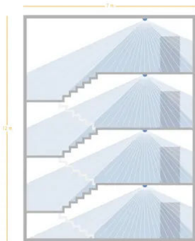
Beispielanwendung Treppenhäuser
