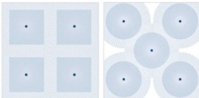
Theben Präsenzmelder sind mit quadratischem, rechteckigem und rundem Erfassungsbereich verfügbar
