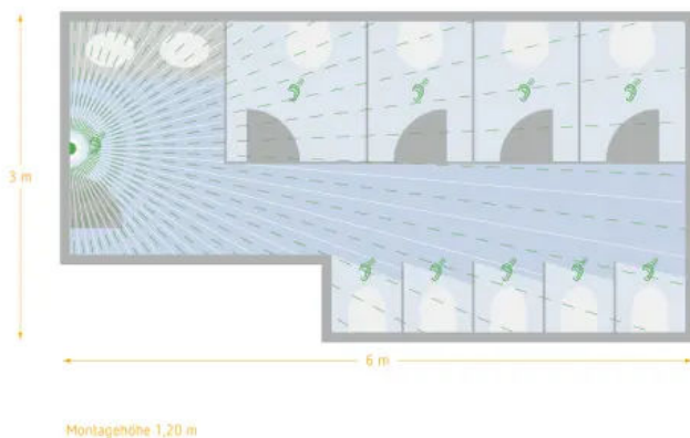
Beispielanwendung Toiletten
