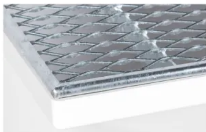
Streckmetall-Kantenschutzrost für Belastungen bis 4,7 kN
