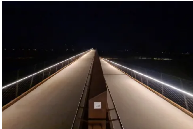
Handlaufsystem LUX GLENDER SAFE - Fußgängerbrücke Buga 2023 in Mannheim | Einseitige symmetrische Beleuchtung der Laufbahn. Ausführung IP65, um ca. 15° gedrehter Handlauf LILLY.
