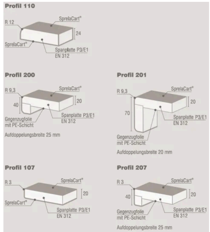
Profile für Decore BASIC und SELECT
