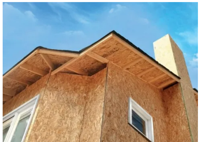
Anwendungsbeispiel OSB Platten
