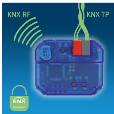
Medienkoppler-TP-RF KNX
