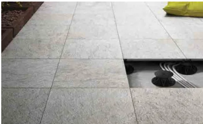
Verlegung auf Stelzenlagern - Die Verlegung auf Stelzlagern ist perfekt für zeitgemäße Bodenbeläge auf Altböden, die zugleich die Unterbringung von Stromkabeln und Rohrleitungen ermöglichen.
