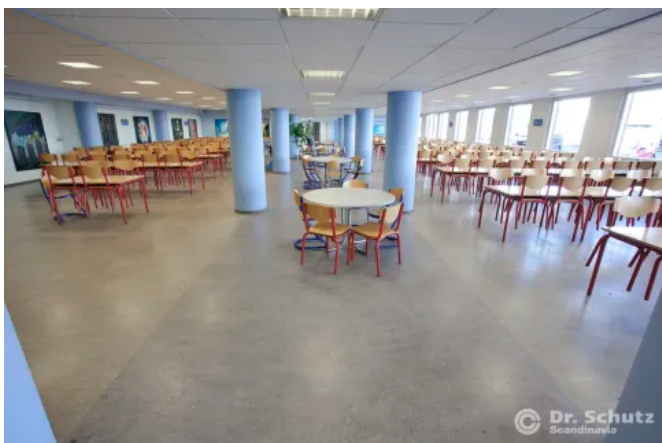
Vorher: TEC Frederiksborg Mensa mit altem, unansehnlichem Boden
