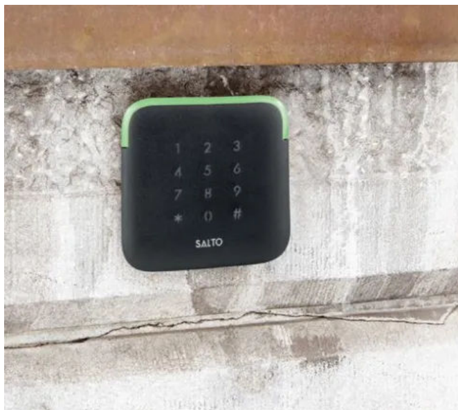
Das wetterfeste Gehäuse schützt die Elektronik (Schutzklasse IP66) für den Außeneinsatz.
